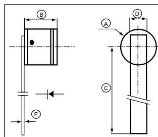
M208e C_b=0.12\text{pF}
