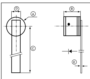
M208d C_b=0.12\text{pF}
