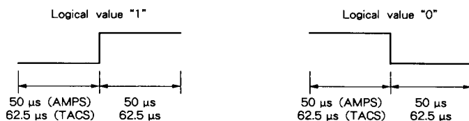
Fig. 1. Manchester code
