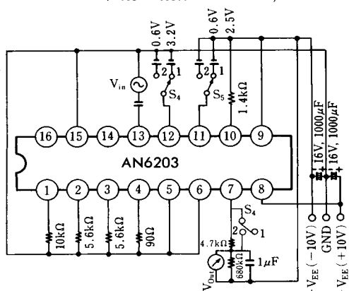
Test Circuit 4 ( V_{R01-4} , V_{L01-3} , V_{I-1-2} , V_{MO} , V_{MOM} )
