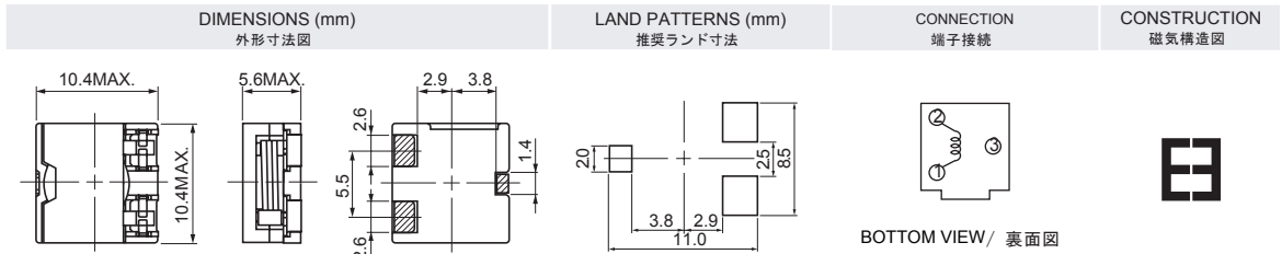
BOTTOM VIEW / 裏面図
