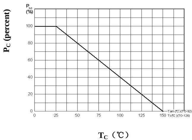
P_C - T_C
