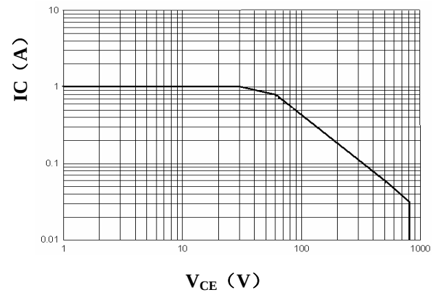
SOA
