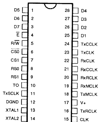
DIP28 : TS68952
