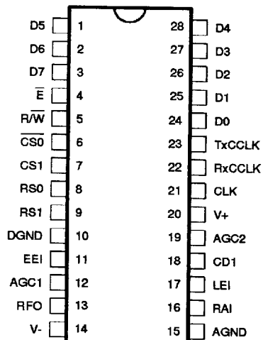
DIP28 : TS68951
