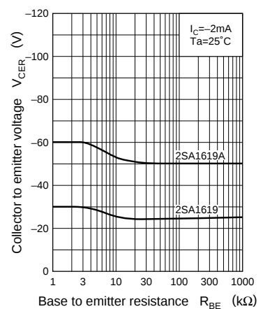
V_{CER} - R_{BE}
