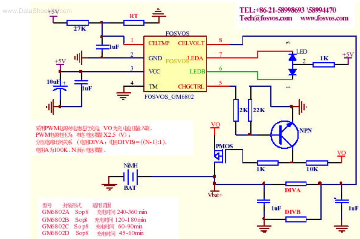
图 5 GM6802 典型应用图
