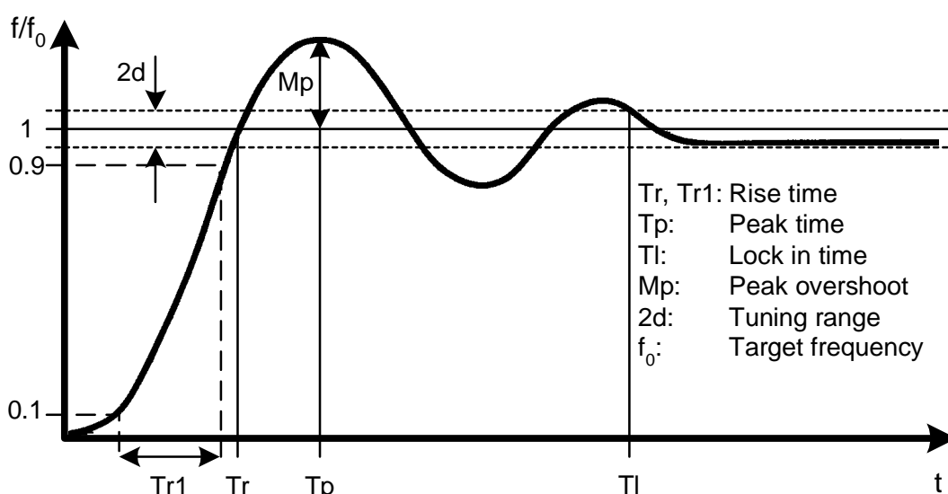
Figure 20 Transient Parameters
