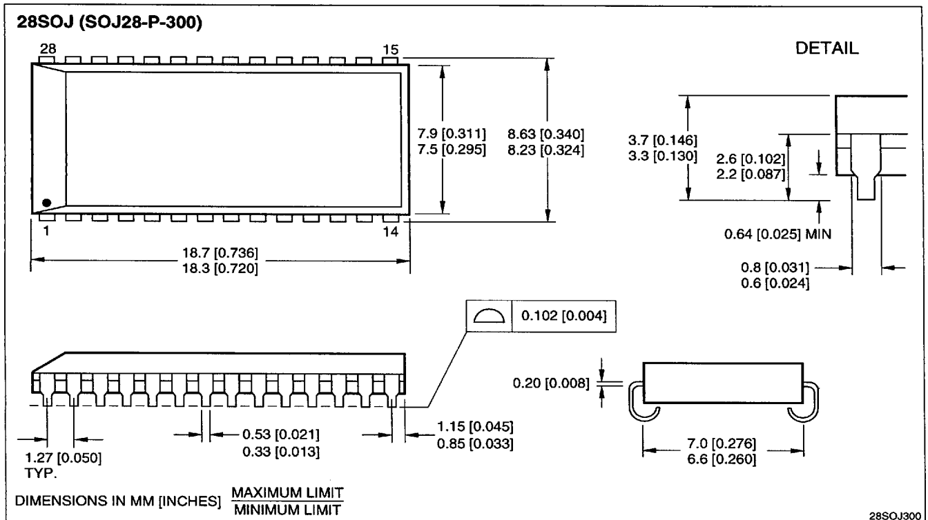
28-pin, 300-mil SOJ
