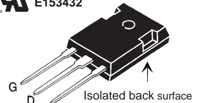
ISOPLUS247™ (IXFR) E153432
