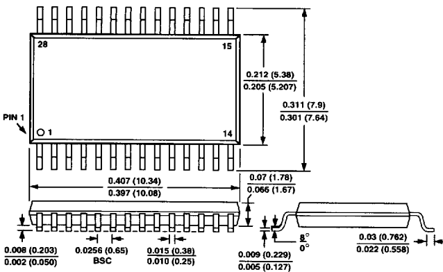
SSOP (RS-28)
