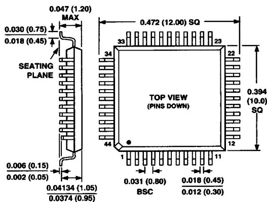
TQFP (ST-44B)
