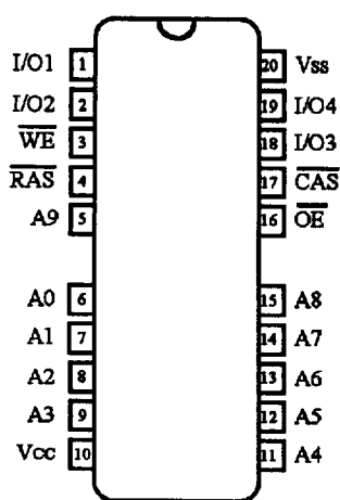
20 (26) SOJ
