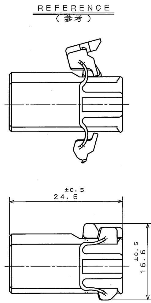
SECT. A-A (SCALE 5:1)
