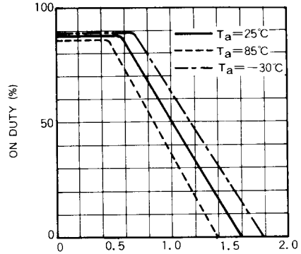
F/B PIN OUTPUT CURRENT
