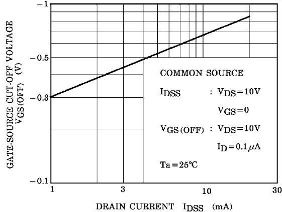
VGS(OFF) - IDSS
