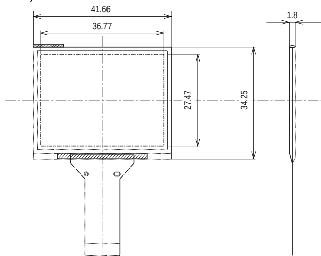
外形図 5107 (unit : mm)
