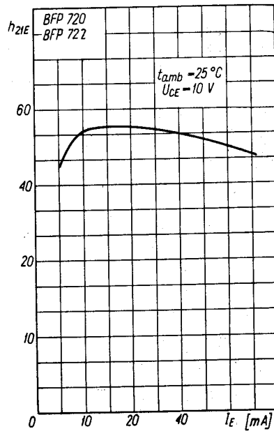
Zależność statycznego współczynnika wzmocnienia prądowego h_{21E} = f(I_E)
