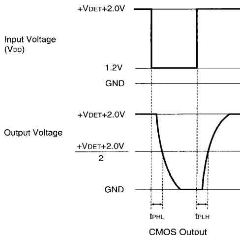
CMOS Output
