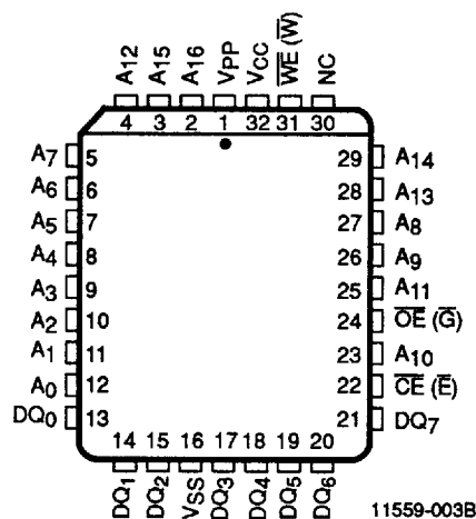
PLCC*
