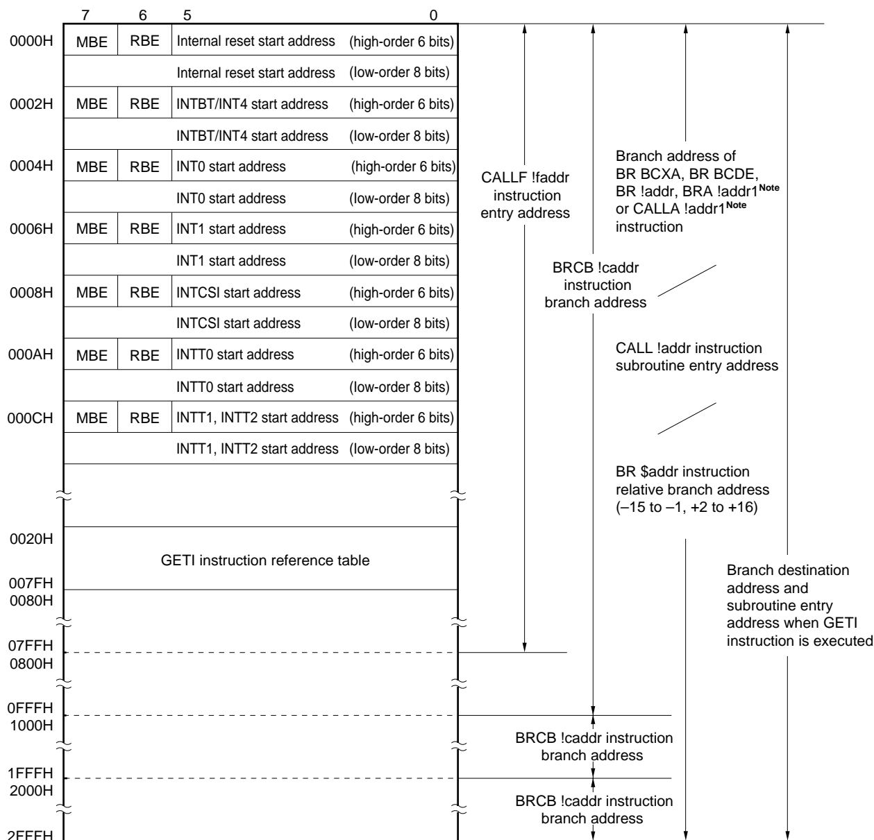
(a) μPD753012A
