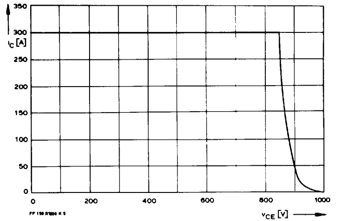
4 Erlaubter Arbeitsbereich in Rückwärtsrichtung. Reverse biased safe operating area. t_{vj} = 125^\circ\text{C} , V_{LF} = V_{LR} = 15\text{ V} , R_G = 8,2\ \Omega
