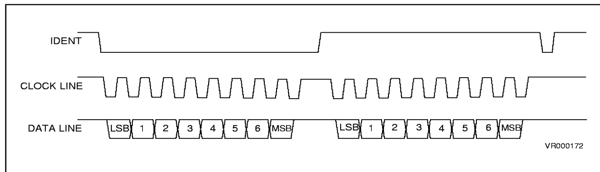
Figure 11-11. IM bus Timing
