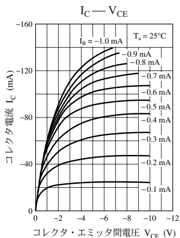
UNR2116 特性図
