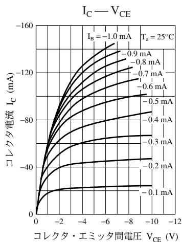
UNR2113 特性図
