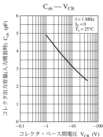
UNR2119 特性図
