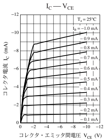
UNR211V 特性図
