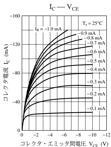
UNR2115 特性図
