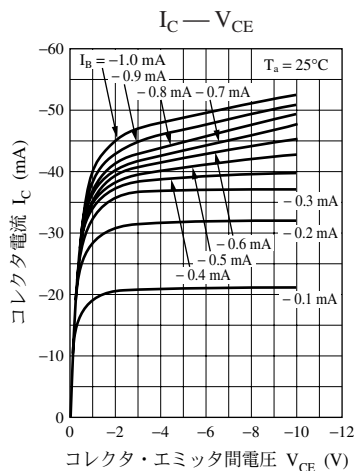
UNR211E 特性図
