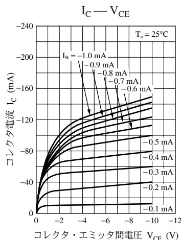
UNR211F 特性図
