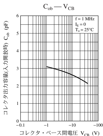
UNR211F 特性図
