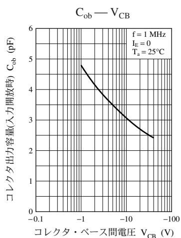
UNR2116 特性図
