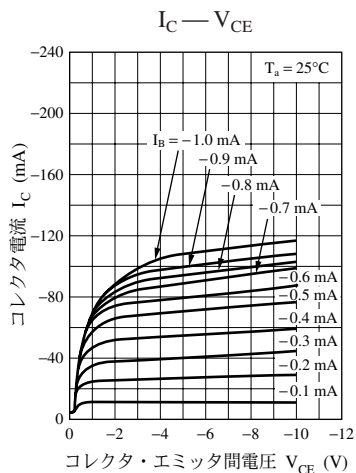
UNR2118 特性図
