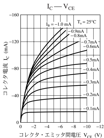
UNR2112 特性図
