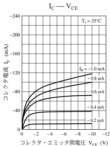
UNR211L 特性図
