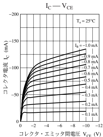
UNR211T 特性図
