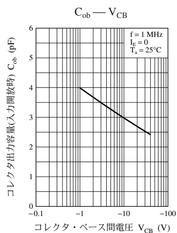
UNR2113 特性図
