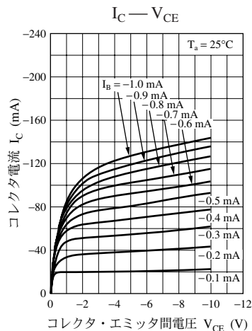
UNR211M 特性図
