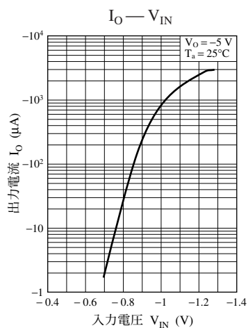
UNR211V 特性図
