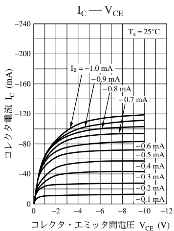
UNR2119 特性図
