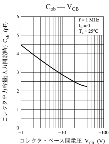
UNR211M 特性図
