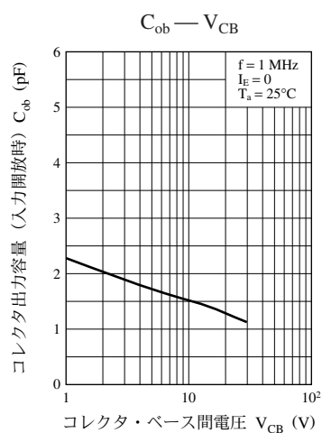
UNR521V 特性図
