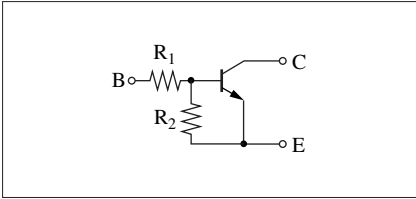
内部接続図
