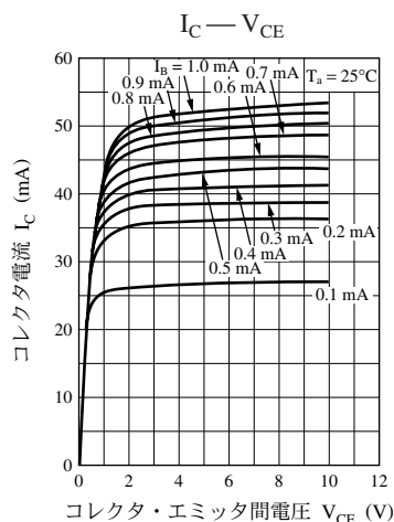
UNR521E 特性図
