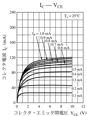
UNR5219 特性図
