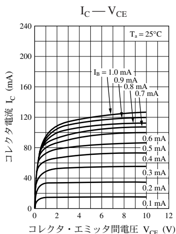
UNR5218 特性図
