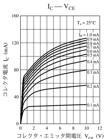
UNR521T 特性図
