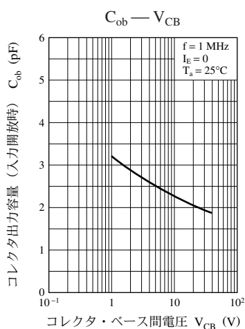
UNR5213 特性図
