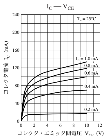
UNR521L 特性図
