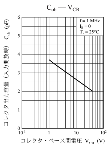
UNR5219 特性図
