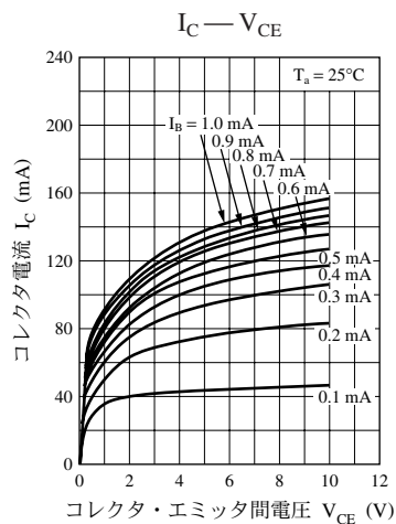
UNR521M 特性図
