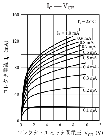
UNR5216 特性図
