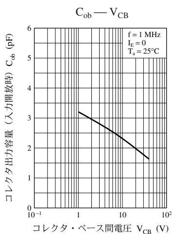
UNR5216 特性図
