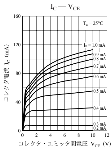
UNR521V 特性図
