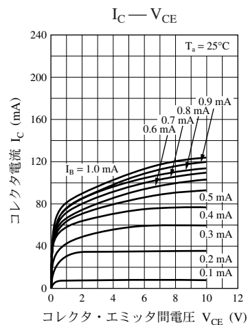
UNR521F 特性図
