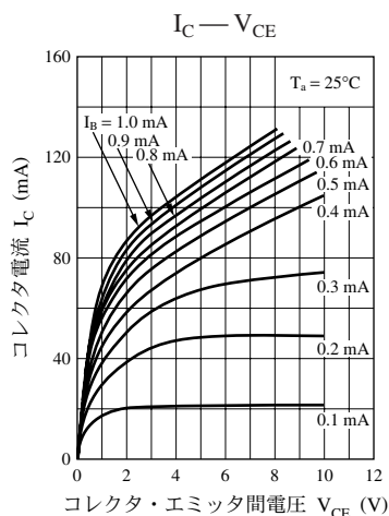
UNR5212 特性図
