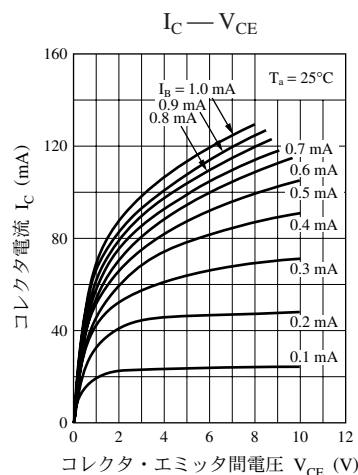
UNR5215 特性図
