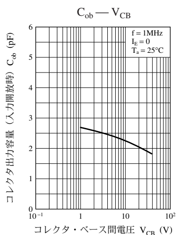
UNR521F 特性図
