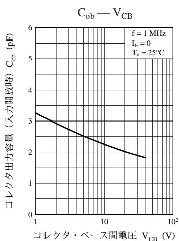
UNR521M 特性図
