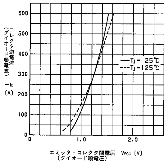
エミッタ・コレクタ間電圧 V_{E0} (V) (ダイオード順電圧) 高速フリーホイーリングダイオード順電圧特性 Forward Voltage of Free Wheeling Diode
