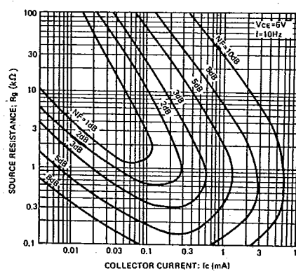
Fig.10 雑音特性 (I)
