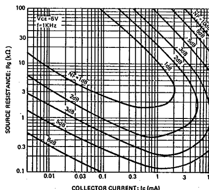
Fig.12 雑音特性 (III)
