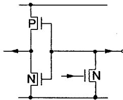
Fig. 4-10: I/O pins SCL, SDA
