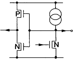
Fig. 4-6: I/O pins PR0, PR1, PR2, FPDAT
