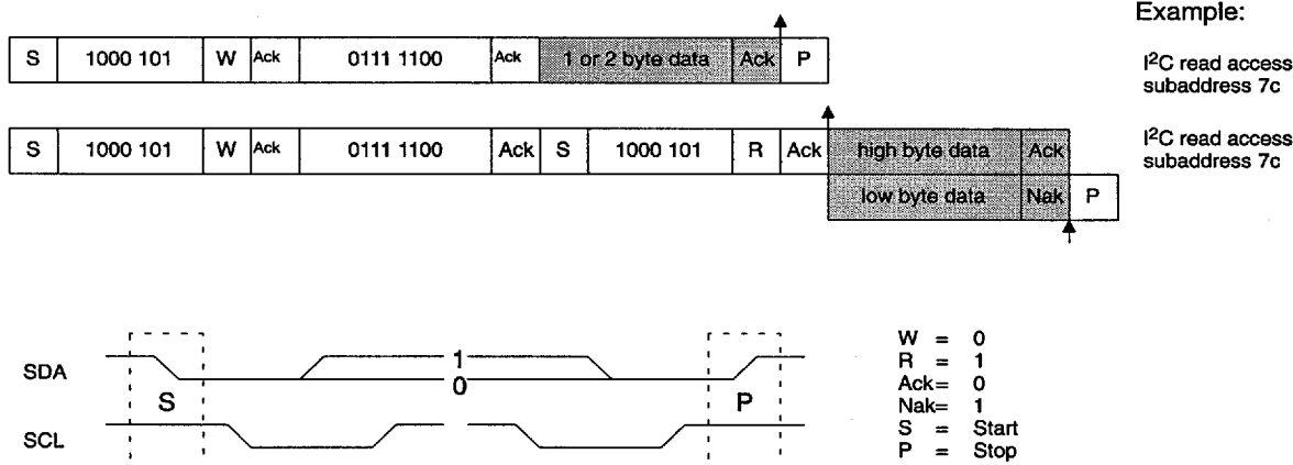
Fig. 3–1: I 2 C-bus protocols
