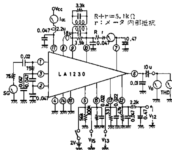
交流特性測定回路
