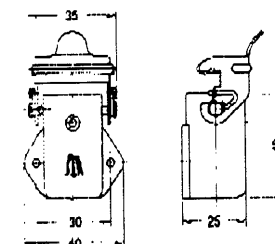
Montageausschnitt/Panel cut-out 20
