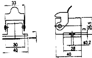
Montageschnitt/Panell cut-out ø 20
