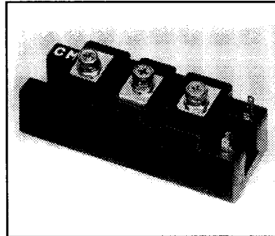
CM50E3Y-24E Chopper IGBTMOD™ E-Series Module 50 Amperes/1200 Volts
