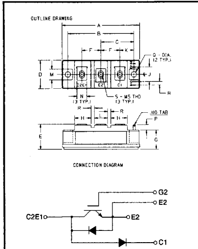
CM50E3Y-24E Outline Drawing
