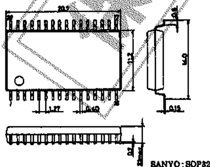
SANYO: SOP32
