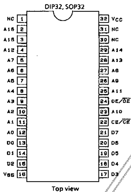
ピン配置図
