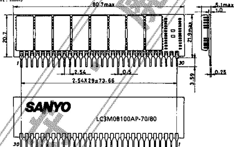
外形図 3184 リードタイプ (unit: mm)
