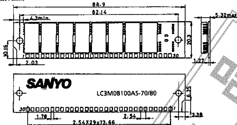
外形図 3183 ソケットタイプ (unit: mm)
