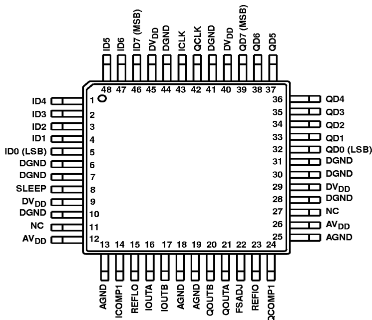
HI5628 (LQFP)
