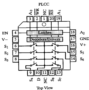
DG528
