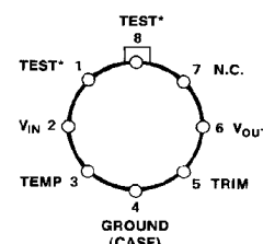
TO-99 (J-Suffix)
