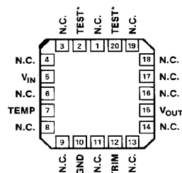
REF-43BRC/883 20-CONTACT LCC (RC-Suffix)
