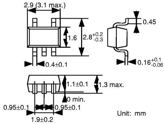
(3) SOT-23-5
