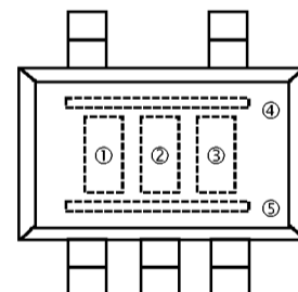
(3) SOT-23-5
