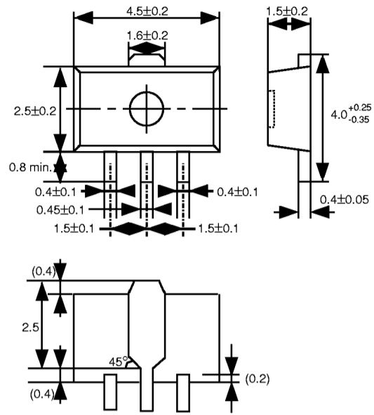
(2) SOT-89-3
