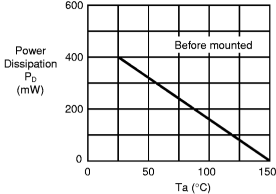
(1) TO-92
