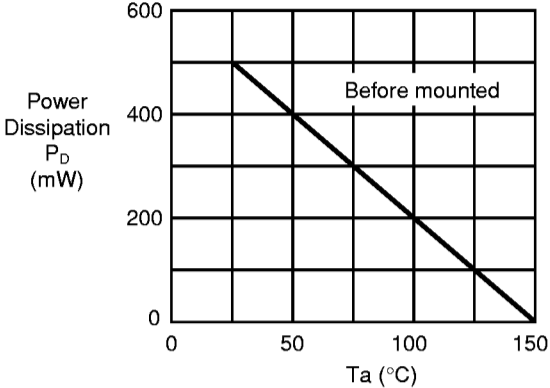
(2) SOT-89-3
