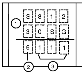
(1) TO-92
