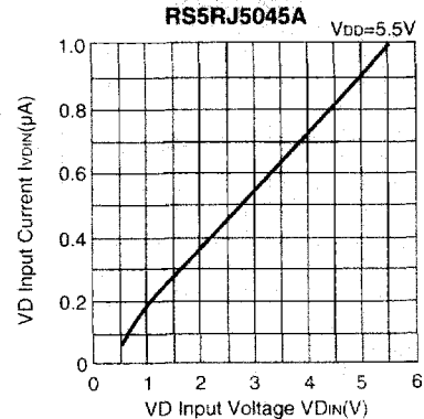
15) VD Input Current vs. VD Input Voltage
