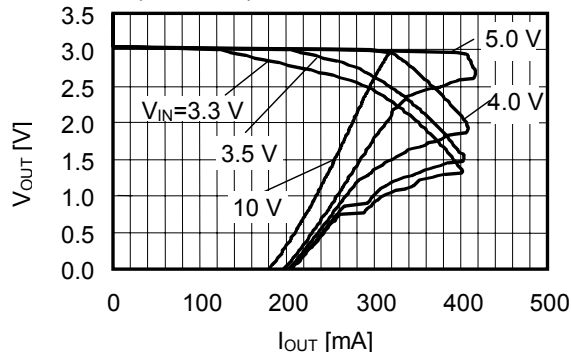
S-L2980A30 (Ta=25°C)
