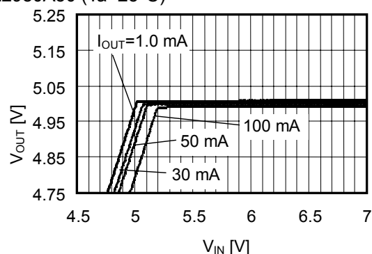
S-L2980A50 (Ta=25°C)
