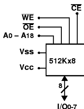
Block Diagram – Flat Package(F3,F16), DIP(P4) & CSOJ(F4)
