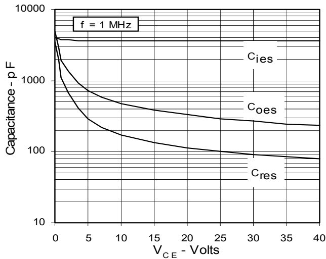
Fig. 15. Capacitance
