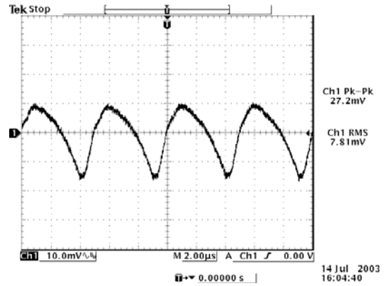
V_{in}=12 V, V_o=1.2 V
