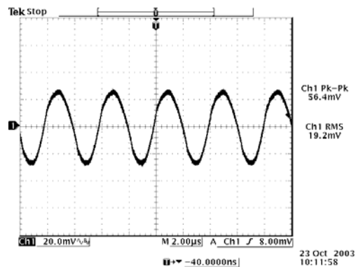
Vin=12 V, Vo=5 V
