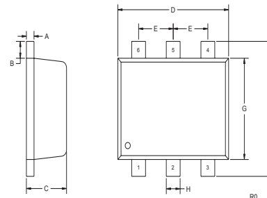
SOT-563
