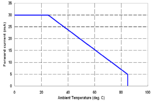
I_F - T_a
