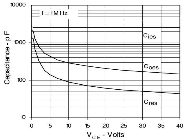
Fig. 12. Capacitance
