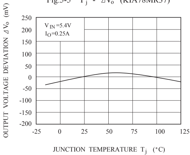
Fig.5-5 T_j - \Delta V_o (KIA78MR37)
