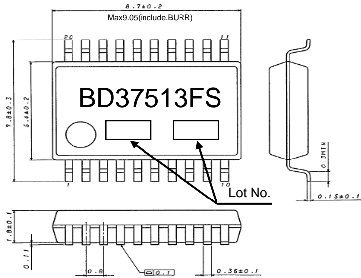
SSOP-A20 (Unit : mm)
