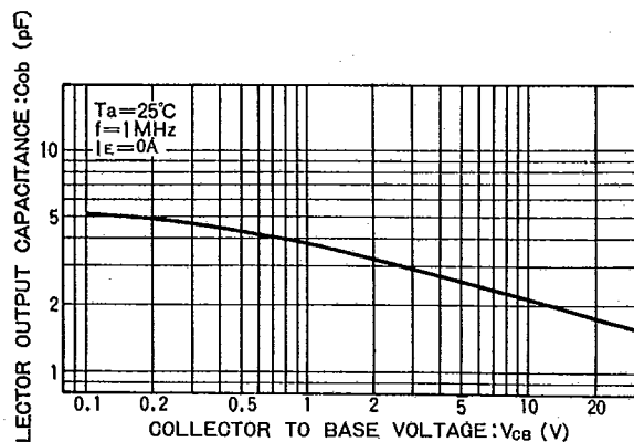
Fig.11 コレクタ出力容量—コレクタ・ベース電圧特性
