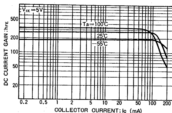
Fig.6 直流電流増幅率-コレクタ電流特性 (II)
