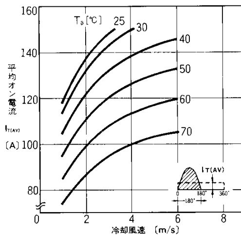
平均オン電流—冷却風速 (正弦波180°導通, 冷却体AL01-20)
