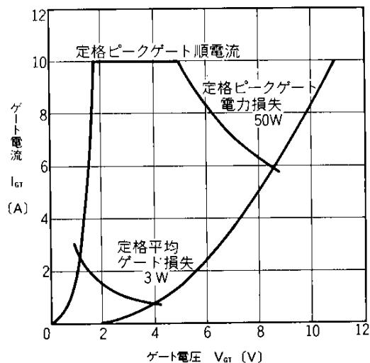
ゲート特性
