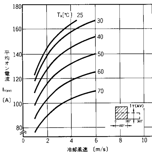
平均オン電流—冷却風速 (方形波180°導通, 冷却体AL01-20)
