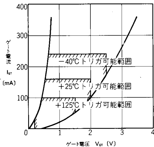
ゲートトリガ特性
