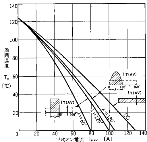
平均オン電流—周囲温度 (冷却体AL01-20, 自冷)
