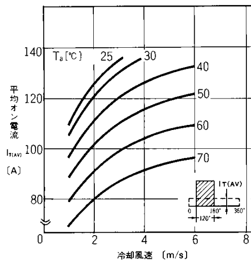
平均オン電流—冷却風速 (方形波120°導通, 冷却体AL01-20)
