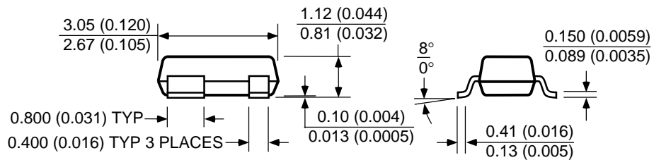
SOT-143 (M4)
